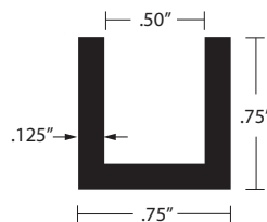
A-774 MF, BK, EA
