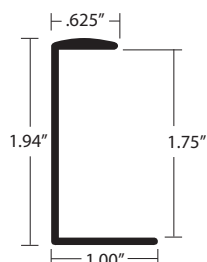
E-146 MF, EA
