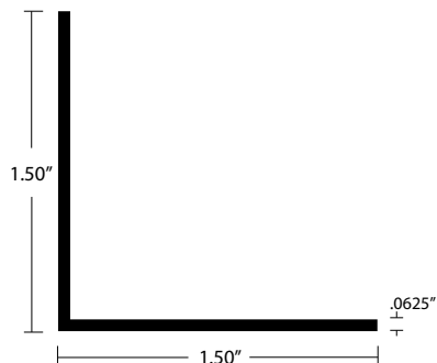
A-1425 MF, BK, EA, MBZ
