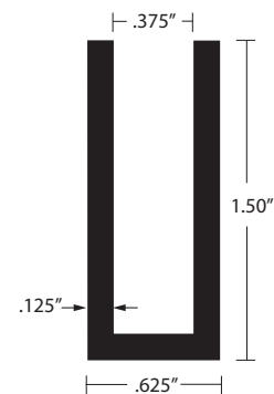
EAM-2763 MF, EA
