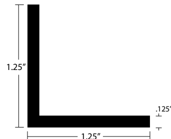
A-1164 MF, EA
